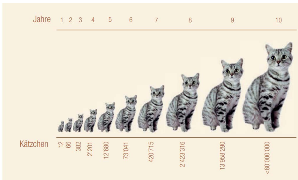
Populationsentwicklung unter idealisierten Bedingungen
