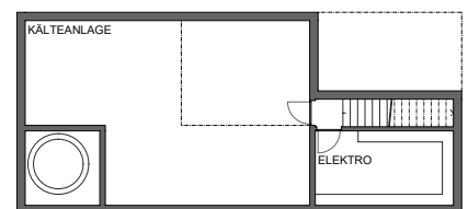
Grundriss Erd- & Untergeschoss Infrastrukturgebäude
