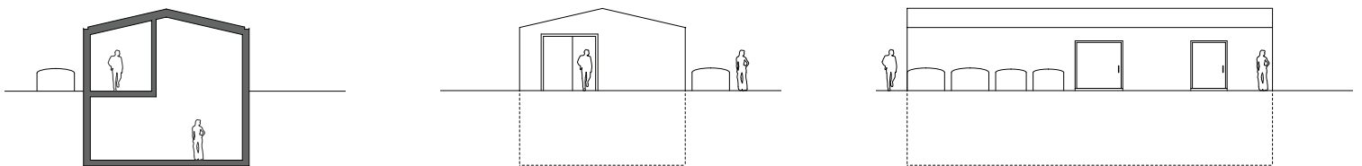
Querschnitt & Längsfassade Infrastrukturgebäude
